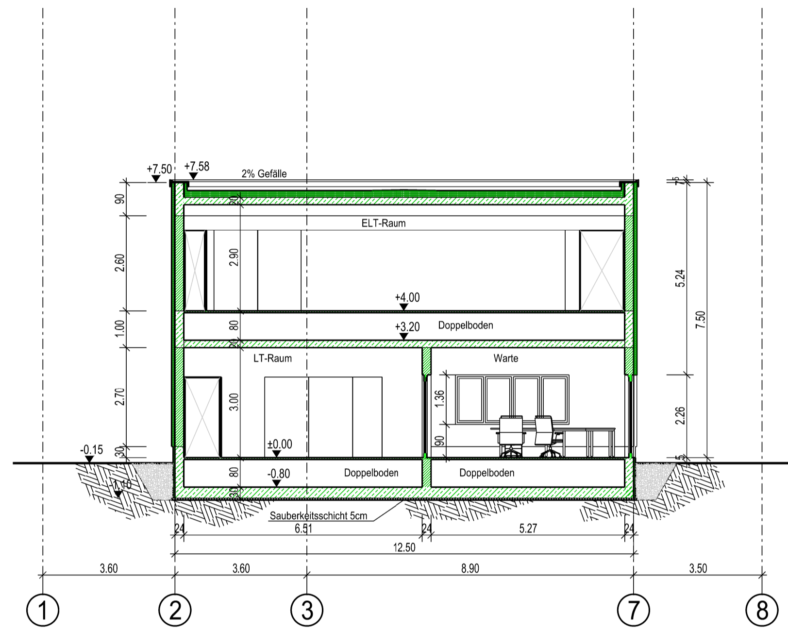
Schnitt B-B
