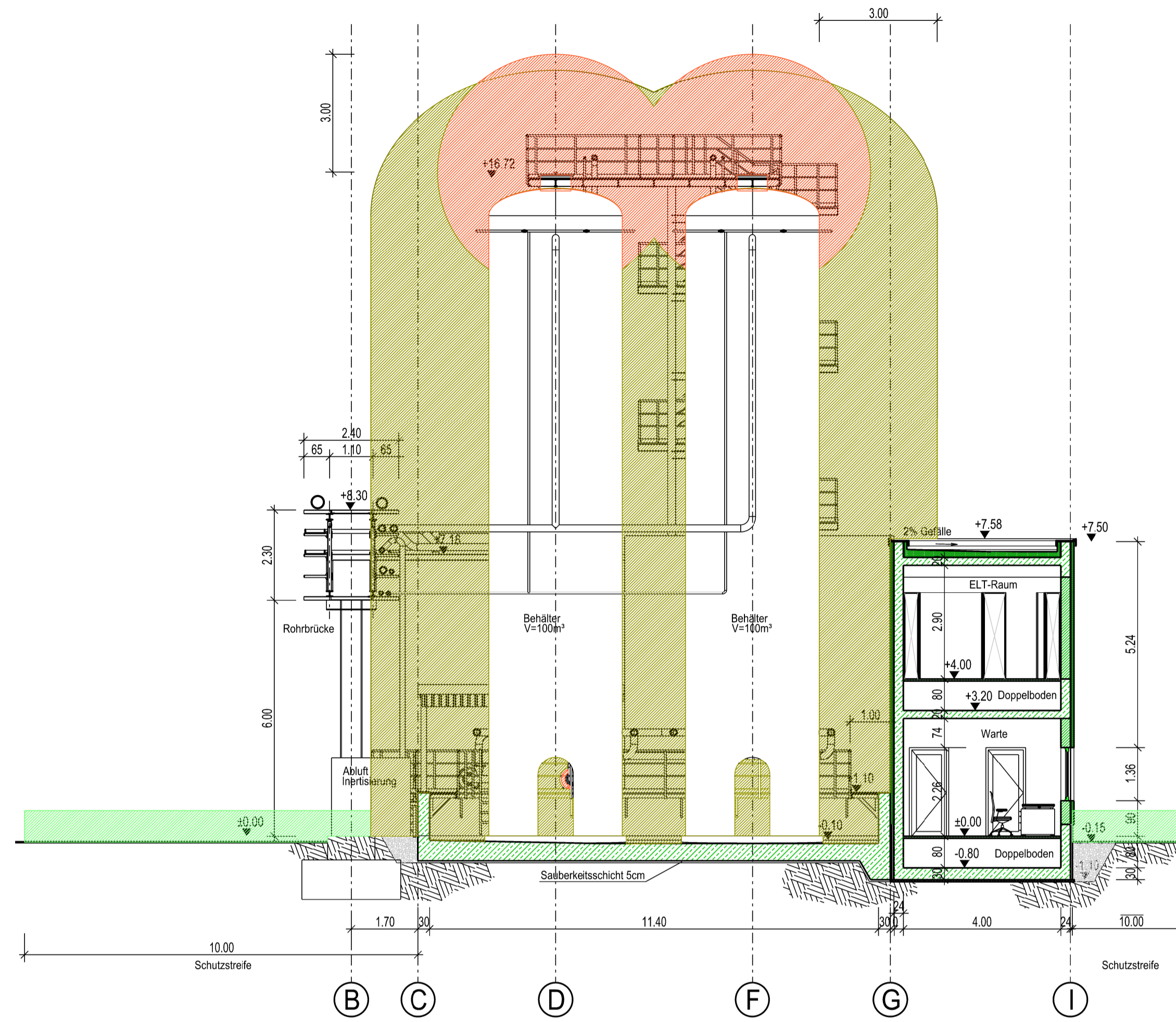
Schnitt C-C
